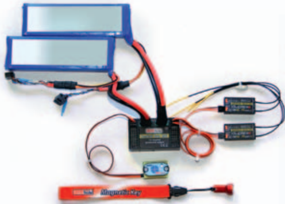
Verkabelung für HV-Servos: Zwei Lipo-Akkus, zwei Satellitenempfänger mit EXBus-Protokoll und Magnetschalter
